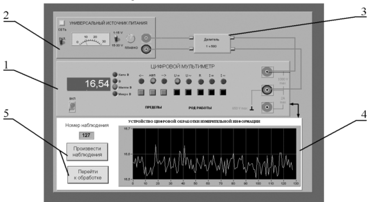
Рис. 1.3.1. Вид модели лабораторного стенда на рабочем столе компьютера при выполнении лабораторной работы № 1.3. (1-электронный цифровой мультиметр, 2-универсальный источник питания, 3-делитель напряжения, 4-индикатор устройства обработки измерительной информации, 5-элементы управления устройством обработки измерительной информации).
